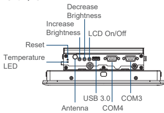
Left I/O
