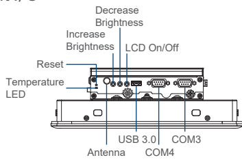
Left I/O
