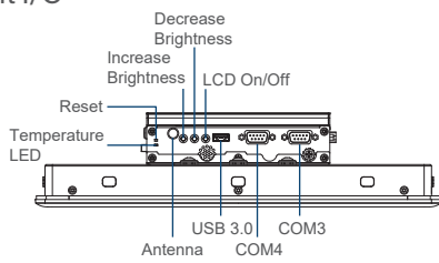
Left I/O
